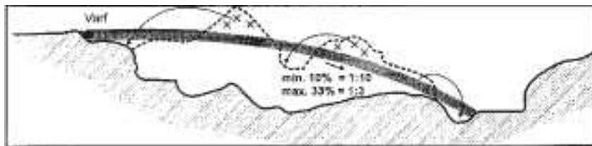
Figura 1.7 - Modelarea formei pentru închidere funcție de amplasament
