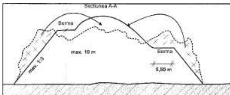
Fig. 1.13a Depozit de deșeuri cu berme 1 - 5 ha - Vedere A - A
