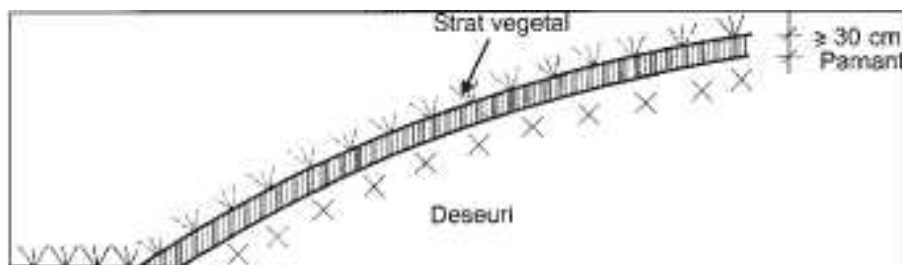
Figura 1.6 - Stratul de acoperire
