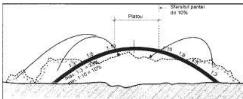
Figura 1.9 Vedere laterală a depozitului
